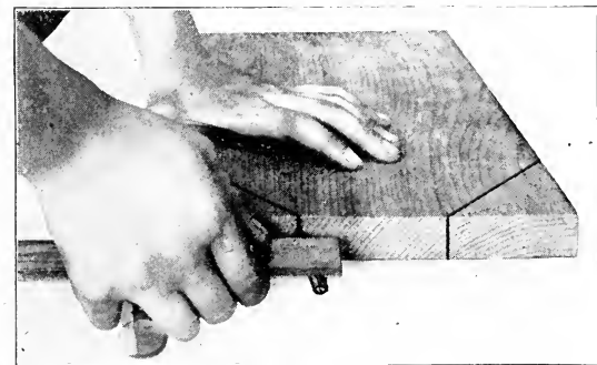
Fig. 146—Gauging Corner
